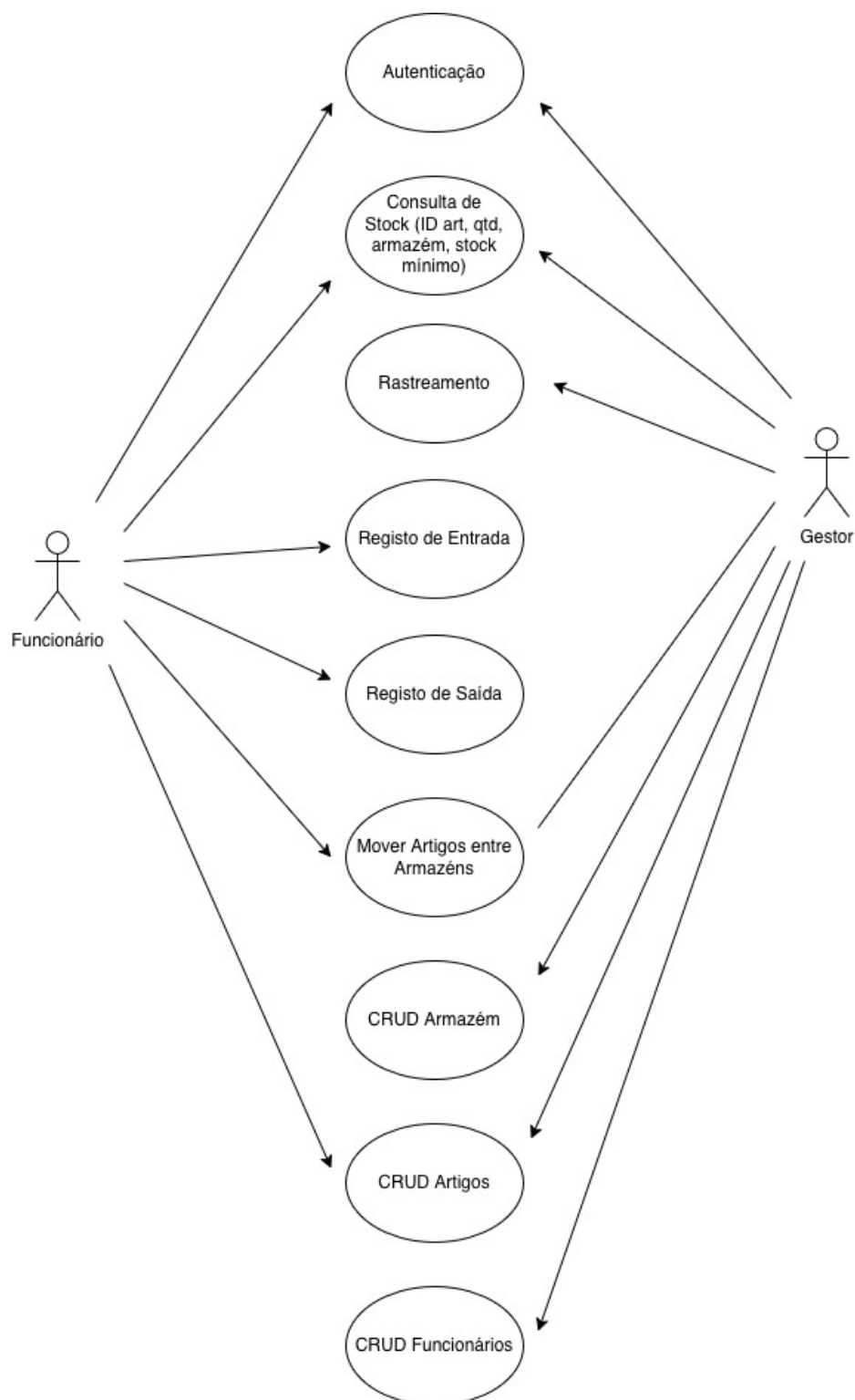
Figura 1- Diagrama de Casos de Uso – Sistema de Gestão de Stock
